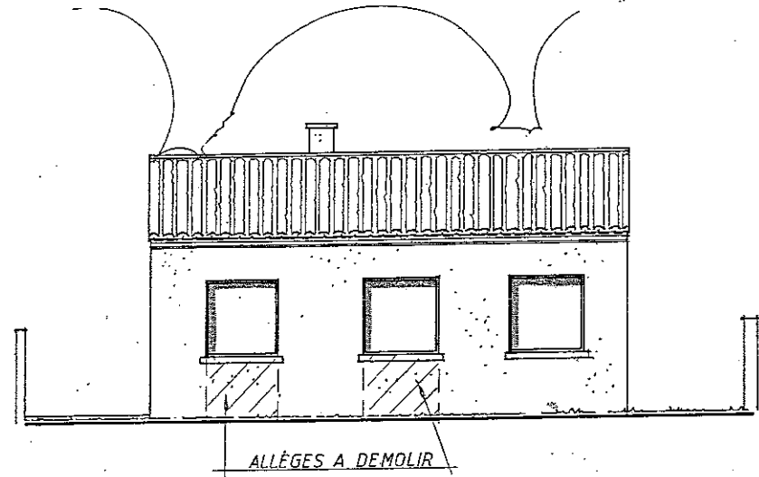
ÉLÉVATION NORD
