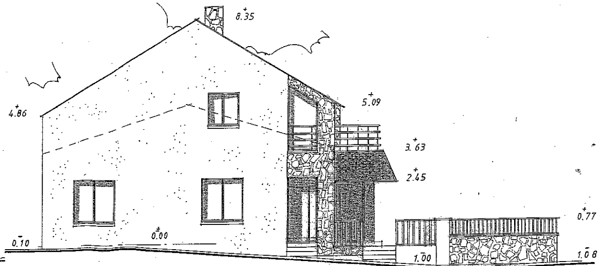
ÉLEVATION OUEST et coupe de niveau sur terrain naturel
